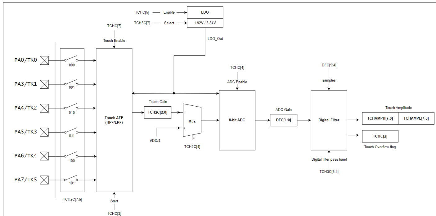
图 23：触摸检测电路的功能方框图
